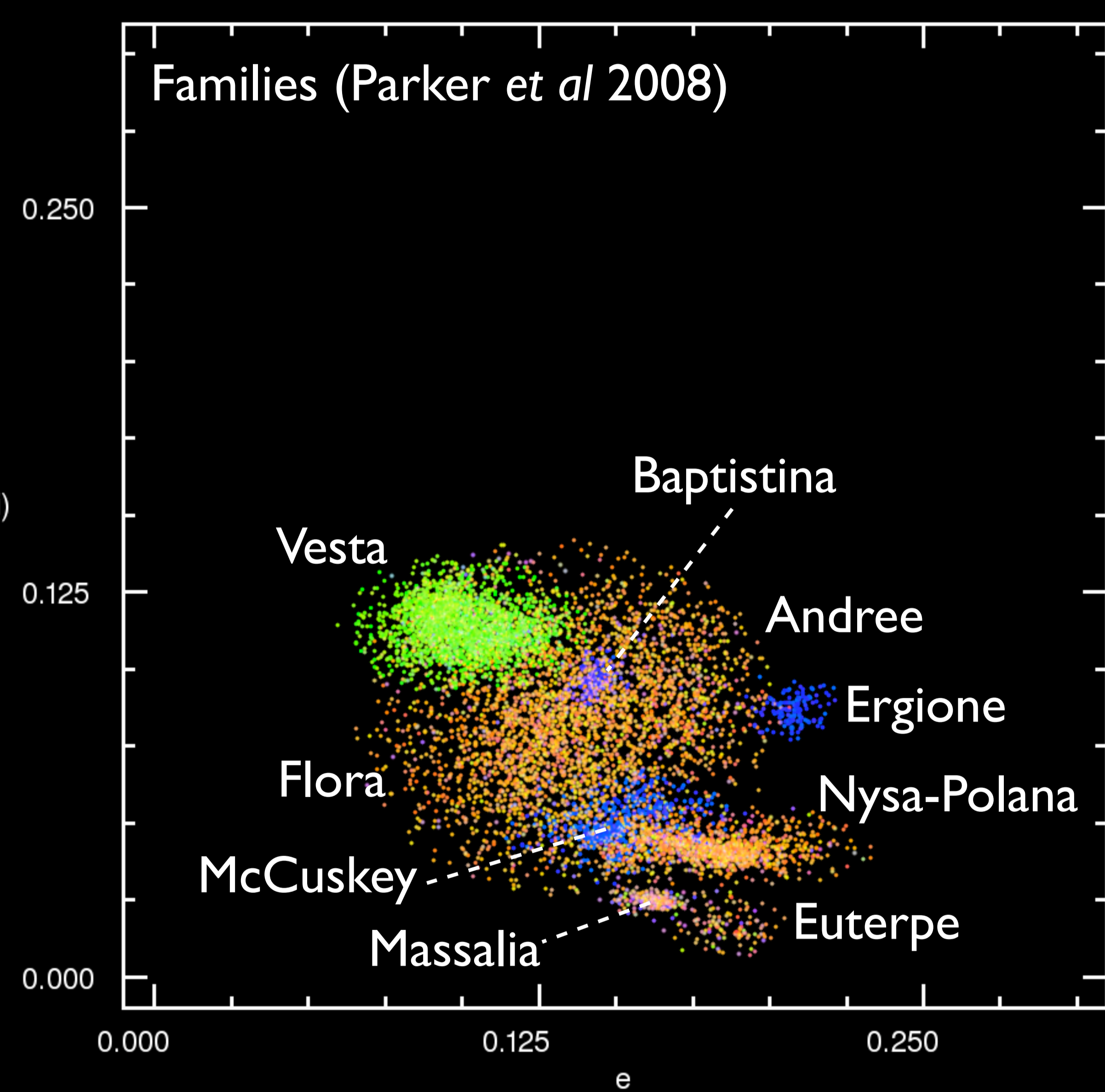
Background (Parker et al 2008)
