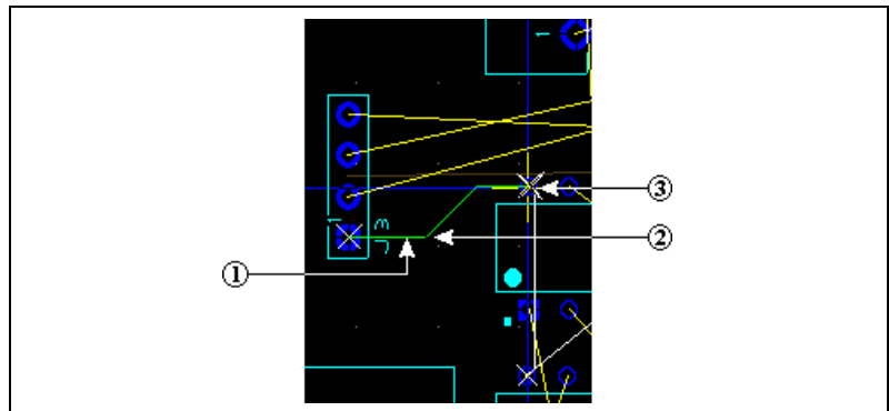
1 Leiterbahn 2 Zum Fixieren der Leiterbahn klicken 3 Endpunkt
