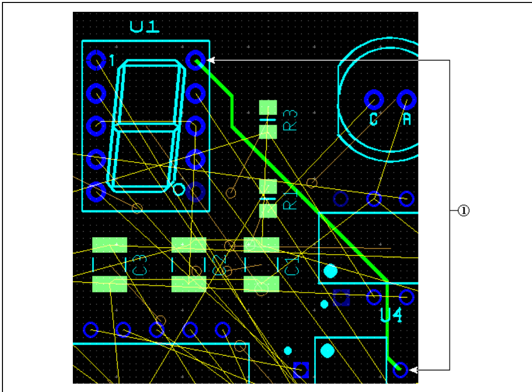
1 Leiterbahnsegmente zwischen Pins
