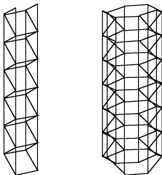
Fig. 7. Acoptic binary ribbons R(3.3.3.4.4)_2 and R(3.3.3.4.4)_4
