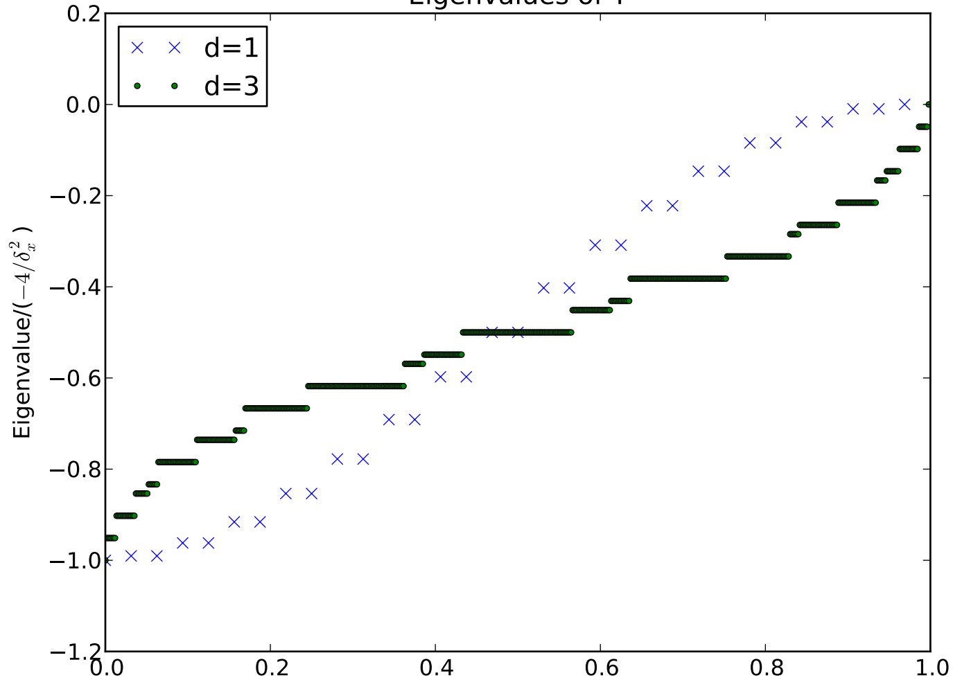
Eigenvalues of T
