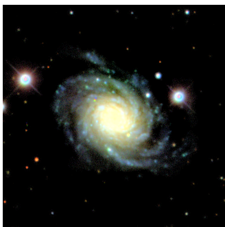
NGC 4030: Sb
