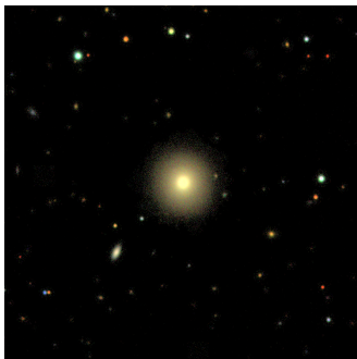
Z 1208.5+0115: E0
