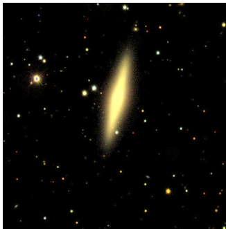
NGC 6010: Sa
