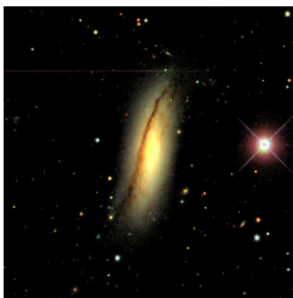
NGC 5719: Sb
