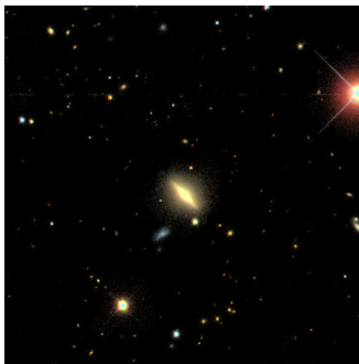
Z 1351.1+0018: E7
