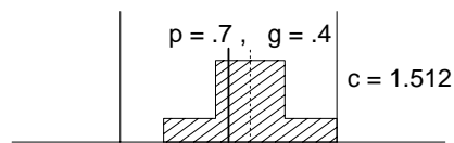
DIN - histogram density
